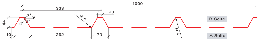
Ausführung: Dach
